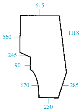
23/4020-27 (D9037, 5136431) Puerta (izq. o drcha) Door (LH-RH)
