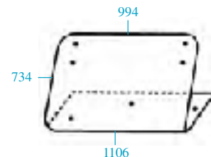
23/4071-15 (D9016, 5124413) Trasero - 7 agujeros Rear - 7 holes
