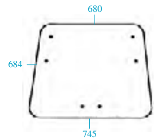
23/4072-73 (D9042, 5136410) Trasero (superior) 6 agujeros Upper rear - 6 holes
