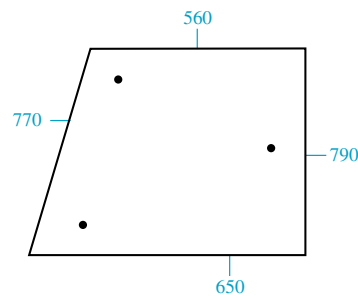
23/4041-7 (D6826, 89861003) Lateral izq. (fijo) Side LH (Fixed)
