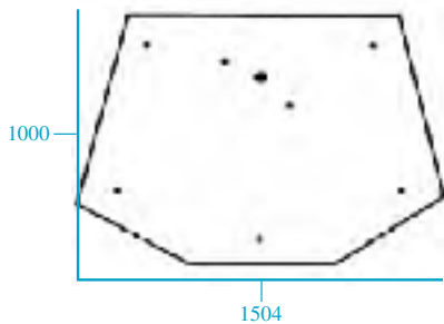
23/4071-28 (D6827, 86002901) Trasero - 8 agujeros Rear - 8 holes
